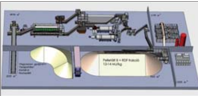
Hulladékfeldolgozó rendszer a körkörös gazdaság és a lokális energiafelhasználás igényei szerint.
